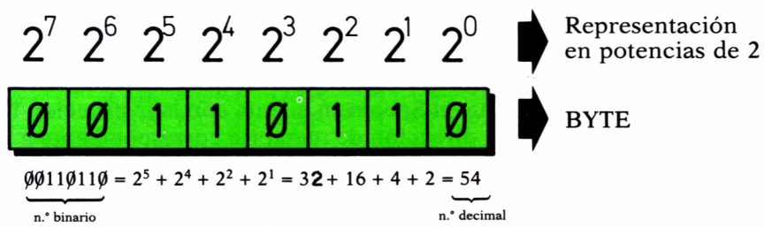
Fig. 4.4. Conversión de sistema binario a decimal.
